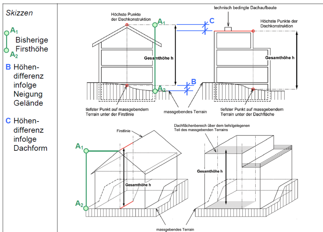
Abbildung 46: Messweise der Gesamthöhe nach IVHB
