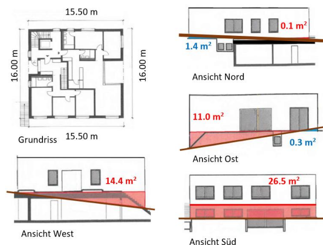
Abbildung 48b: Messweise der Unterniveaubauten nach IVHB und kant. Praxis
