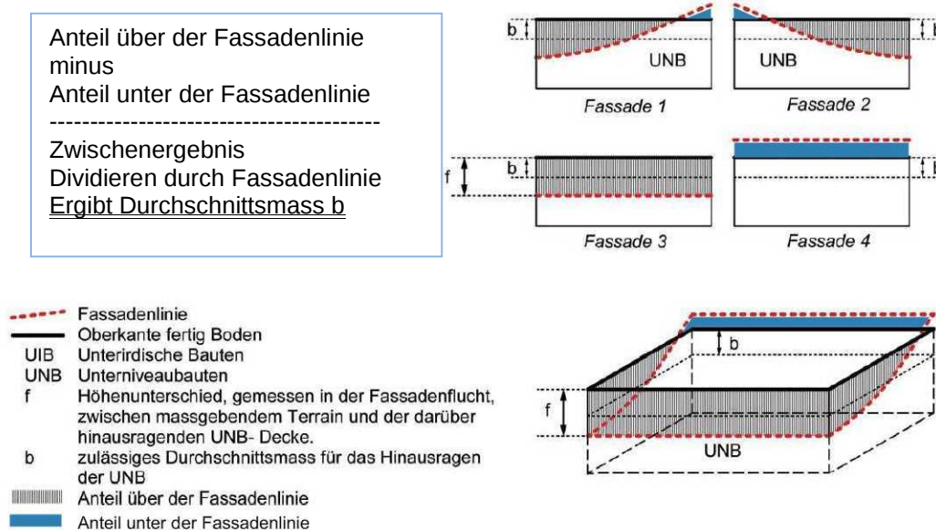
Abbildung 48a: Messweise der Unterniveaubauten nach IVHB
