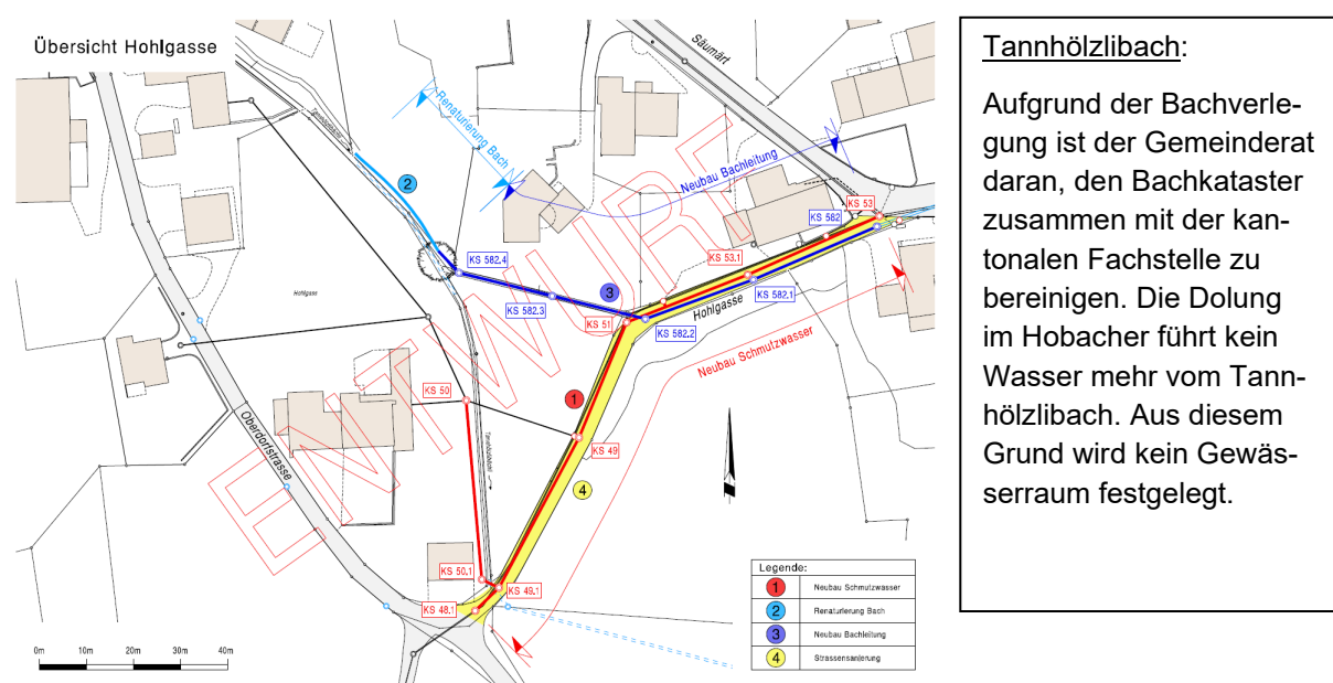
Abbildung 52: Ausschnitt Bachverlegungsprojekt Tannhölzlibach
