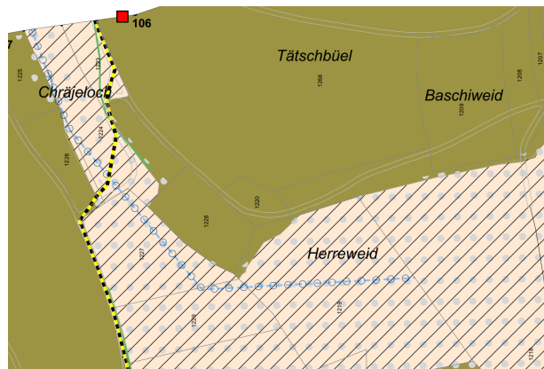
Abbildung 54: Drainageleitung Chräjeloch
