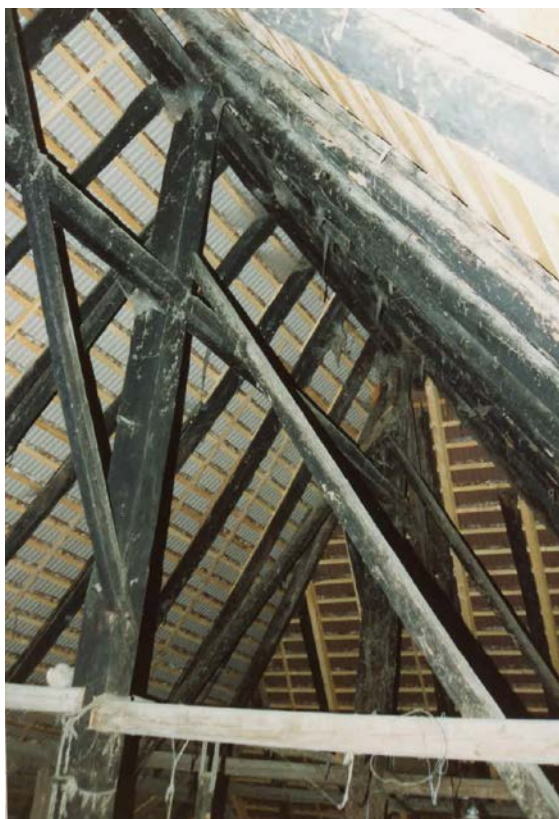
Rauchgeschwärzte Hochstud-Dachkonstruktion (Kurzinventar 1992)
