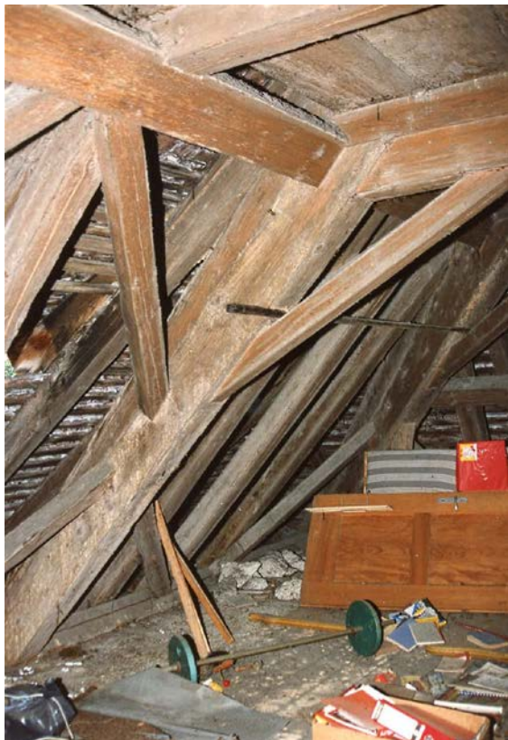
Dachkonstruktion mit liegendem Stuhl (Kurzinventar 1992)
