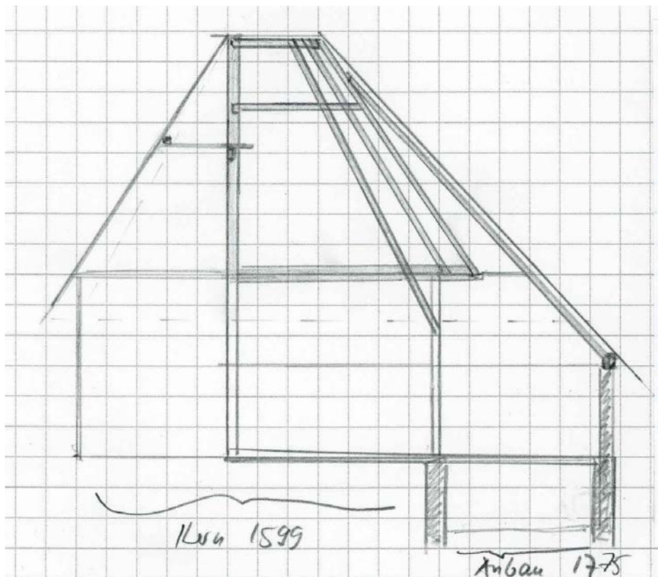
Längsschnitt der Einer-Hochstudkonstruktion (Kurzinventar 1992)
